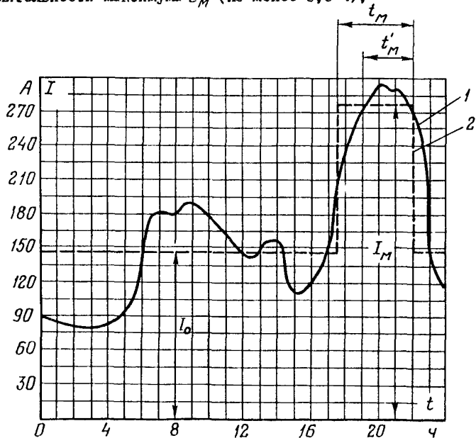
Рис.П 5.1. Приведение суточного графика нагрузки к двухступенчатому виду:
