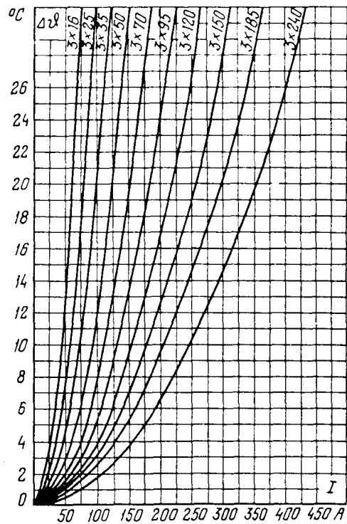
Рис.П7.5. Разность температур между бронентами (оболочкой или шлангом) и алюминиевыми жилами кабелей 10 кВ, находящихся в эксплуатации от 10 до 25 лет
