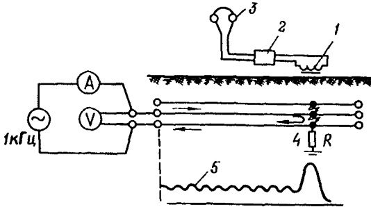
Рис. П20.2. Определение места повреждения индукционным методом:
