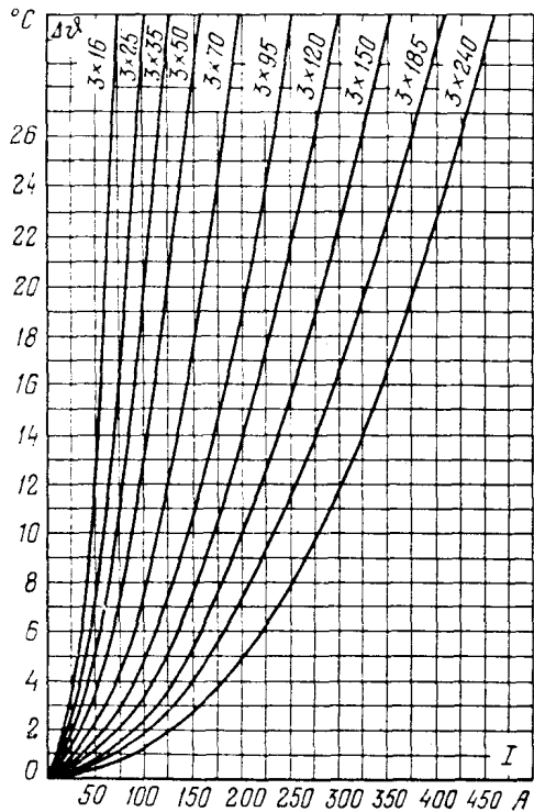
Рис.П7.4. Разность температур между бронентами (оболочкой или шлангом) и алюминиевыми жилами кабелей 6 кВ, находящихся в эксплуатации от 10 до 25 лет
