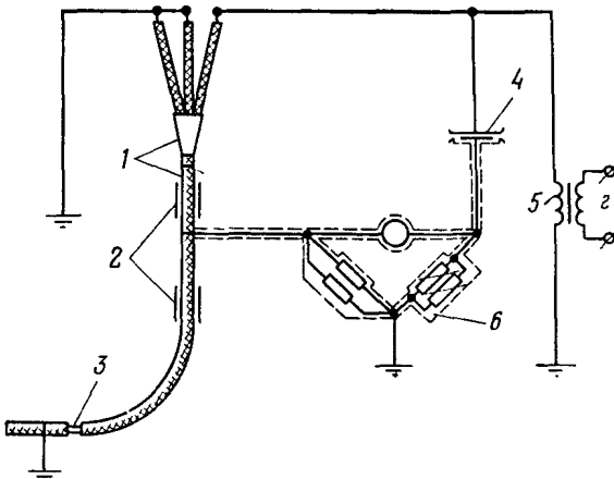
Рис. П7.1. Схема измерений диэлектрических потерь в изоляции вертикальных участков линий:
